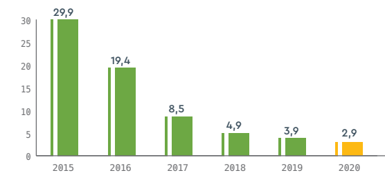
ДИНАМИКА ПАРОНЕФТЯНОГО ФАКТОРА, т пара на 1 т нефти
